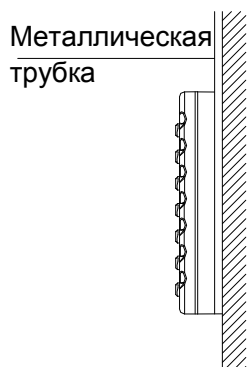
Рис. 2 Открытая установка кабеля
