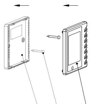
Рис. 4 Схема установки
